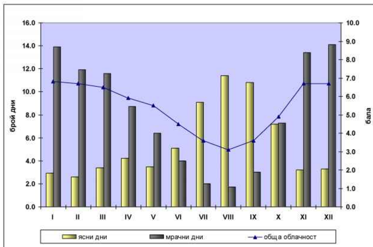
Фигура 1.4.2-2 Месечен брой на ясните и мрачните дни по общ облачност за ст. Шумен.
